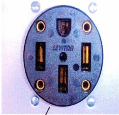
50 amp 125/250 volt 4 wire receptacle (common type)
